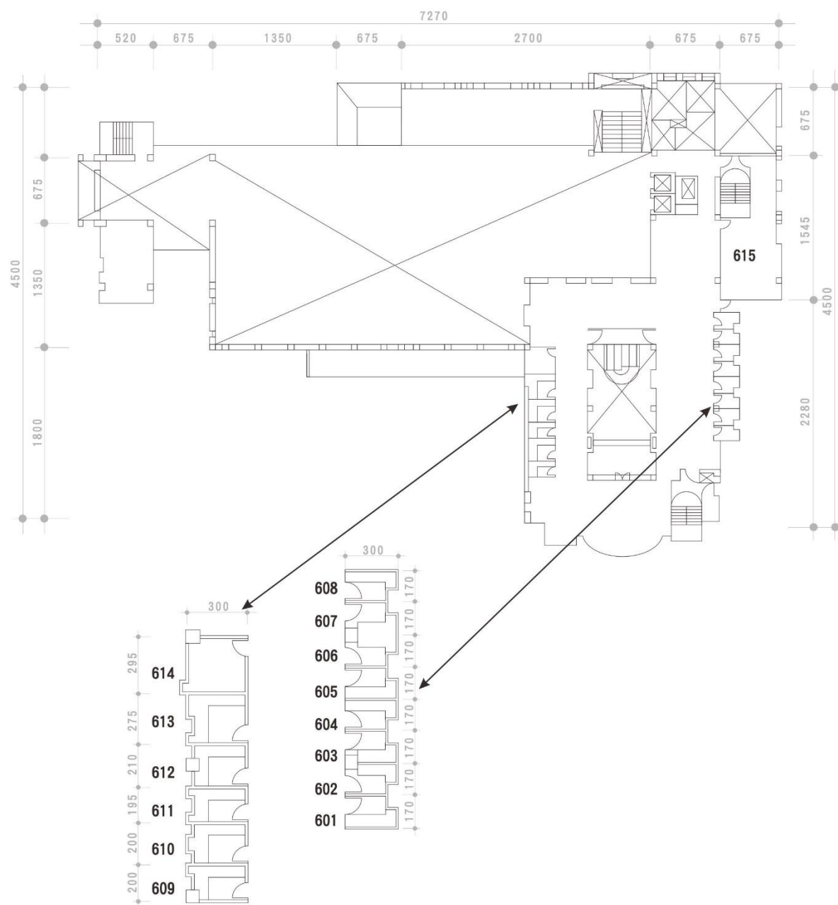
圖書館六樓平面圖
