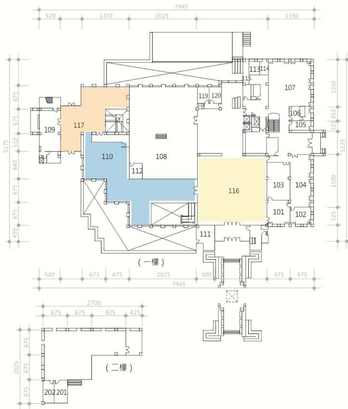
圖書館一、二樓平面圖
