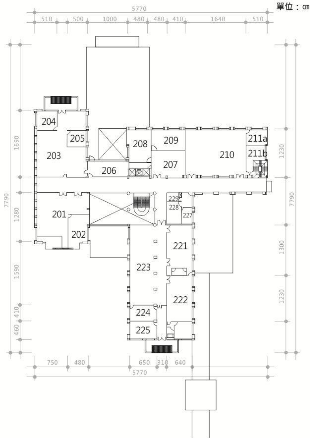
行政中心二樓平面圖
